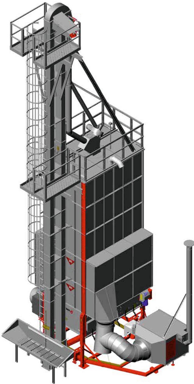
Изделие на рисунке оснащено элеватором с прямым приводом (E), который спроектирован для высоких конструкций силосных бункеров.
