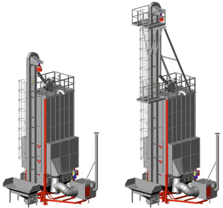
С 320 E, элеватор с прямым приводом
